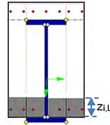
Stützenquerschnitt
