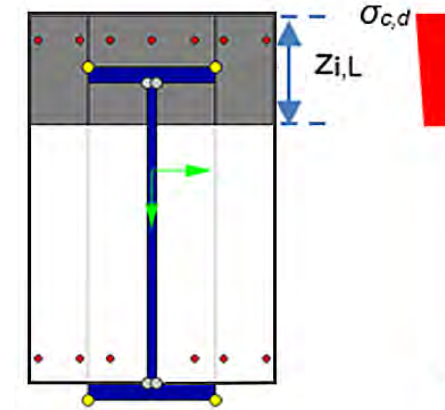
Feldquerschnitt
