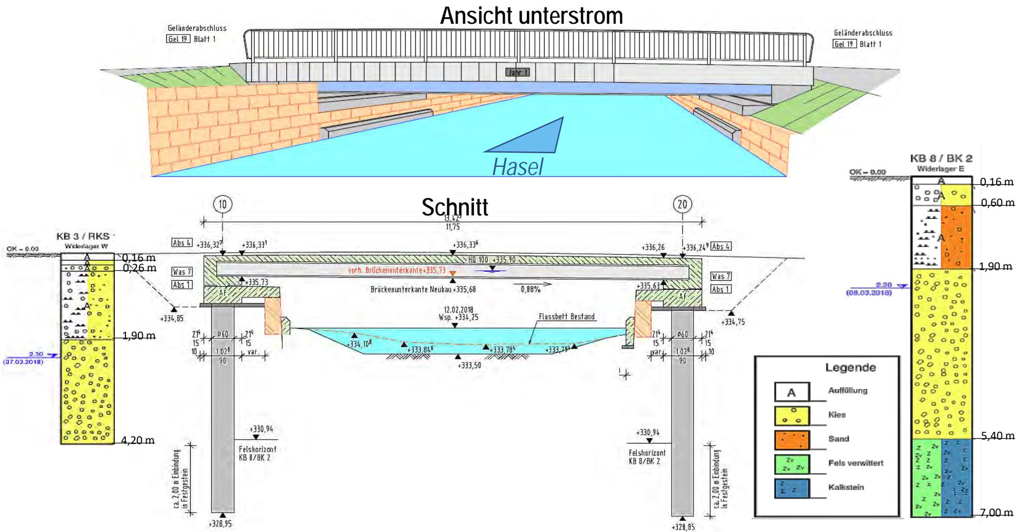
Systemabmessungen der kommunalen WIB-Brücke über die Hasel in Dillstädt/Schwarza
